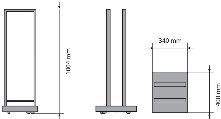
HOUTBLOKKENKARRETJE
